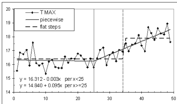
Figura 4: analisi di discontinuità piecewise e flat steps a confronto per le temperature massime medie annue nel periodo 1956-2004
